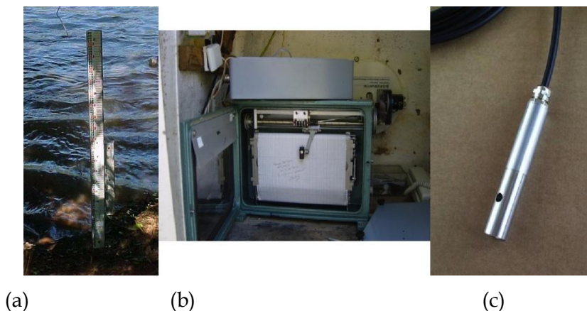
Figura 5.7. a) Limnómetro, b) limnógrafo, c) sonda de nível
