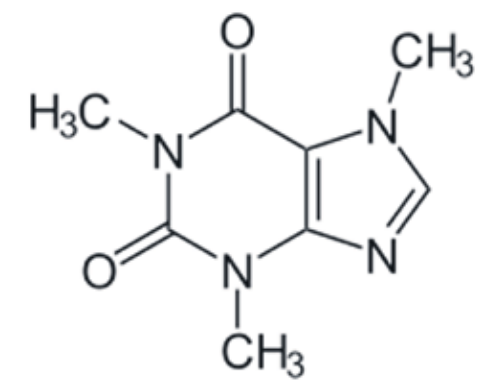
Estrutura molecular da cafeína
