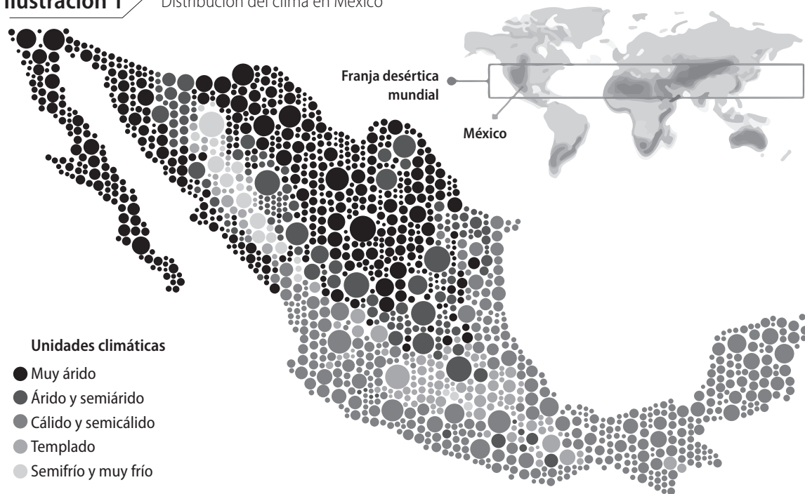
Ilustración 1 Distribución del clima en México
