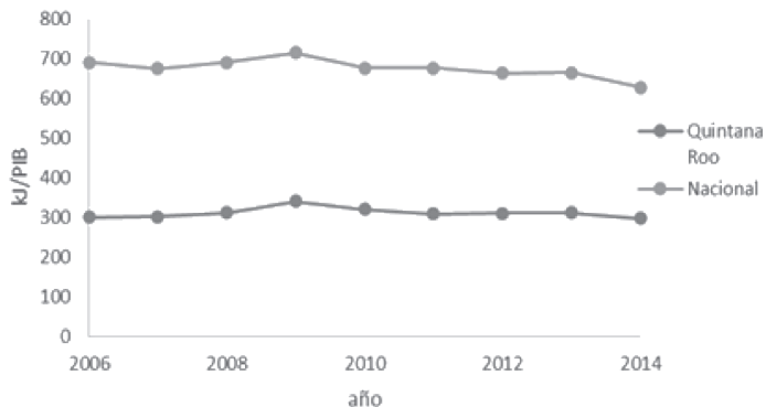
Figura 13. Comparación de los indicadores nacional y estatal del consumo de energía/PIB en el sector industrial
