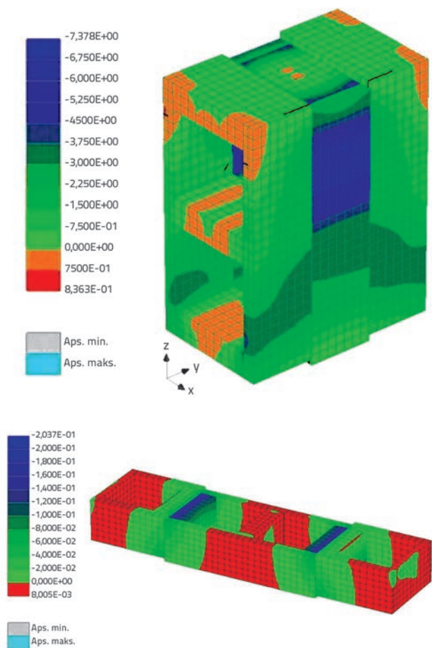
Slika 12. Normalna naprežanja u šupljem opečnom zidnom elementu za smjer opterećivanja usporedno s horizontalnim (gore) i vertikalnim sljubnicama morta (dolje), dimenzije u N/mm 2
