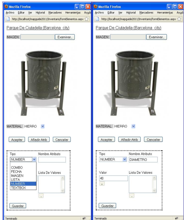
Figura 4.6 Añadir atributo (ejemplo 1), panel para insertar los valores
