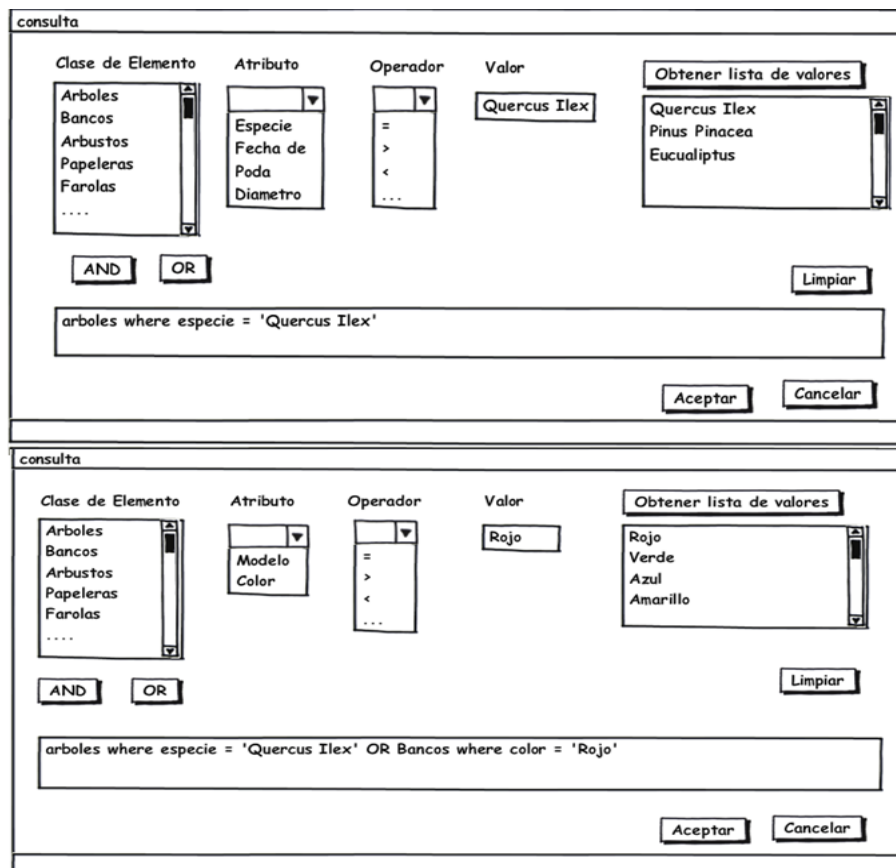
Figura 3.7 Formulario de consulta
