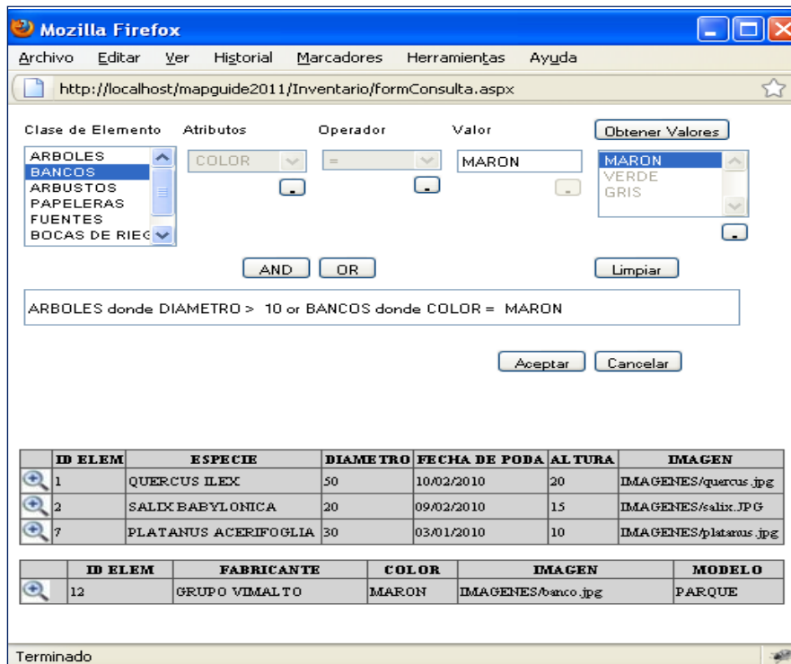
Figura 4.11 Ejemplo, formulario de consulta
