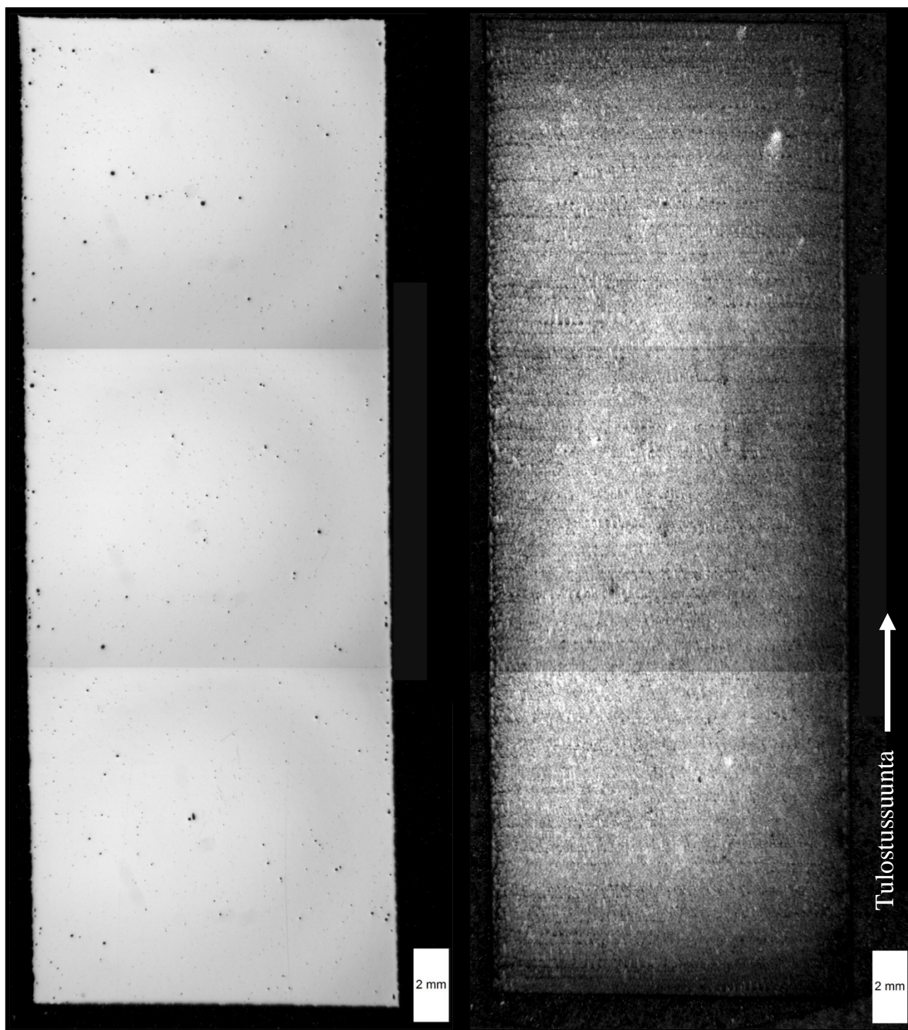
Kuva 2.1. Tulostustilainen Inconel 718 näyte a) ennen syövytystä, b) syövytyksen jälkeen.
