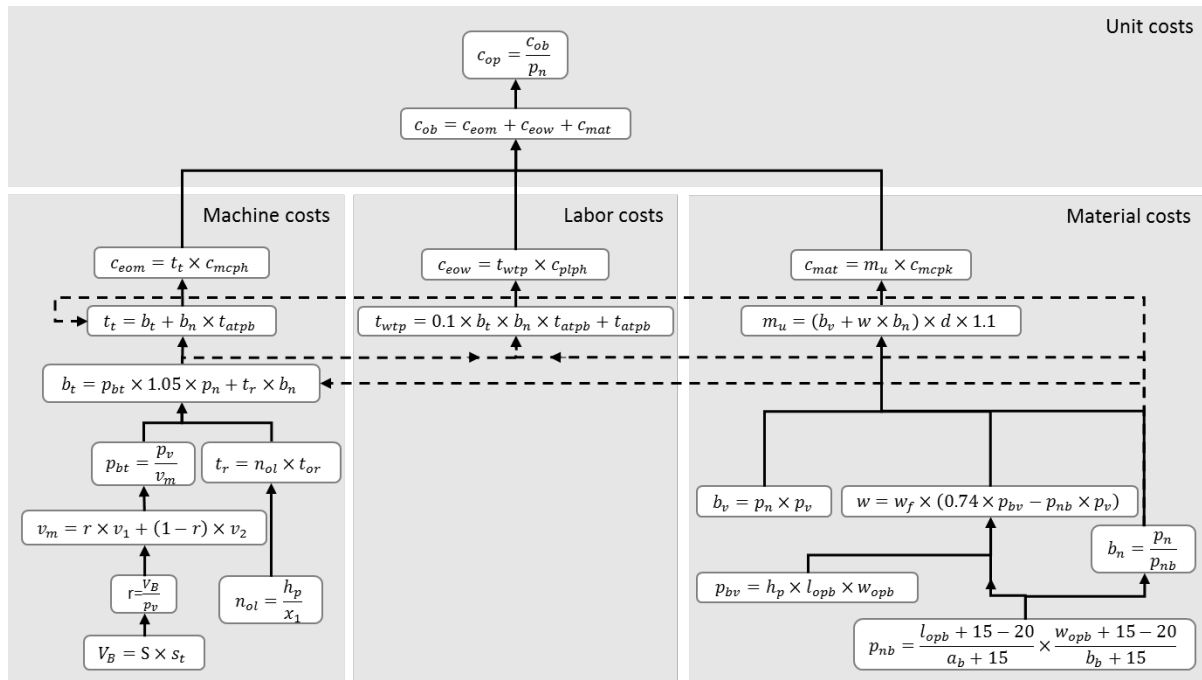
Kuva 4. Metallien jauhepetitekniiikan kustannustyyppikohtaiset funktiot. 2
