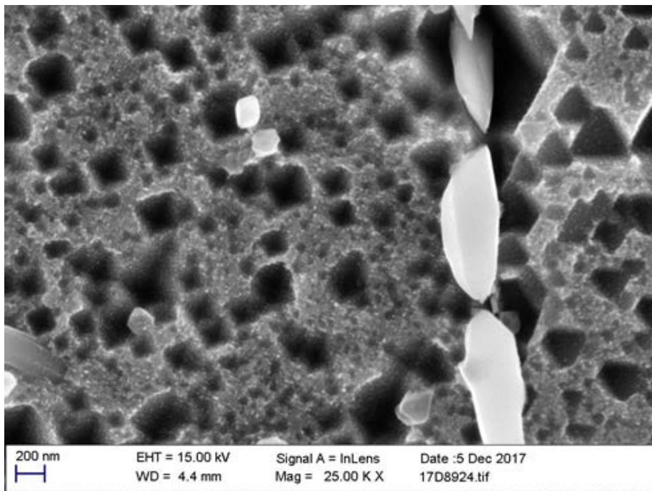
Kuva 3.6. 3D-tulostettu ja lämpökäsitelty (Jännitystenpoisto + HIP + Liutushehkus + Erkautuskarkaisu) Inconel 718 SEM kuva 25000x suurennoksella.
