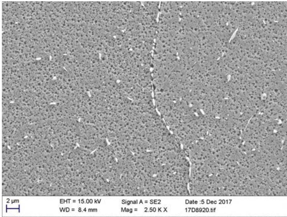
Kuva 3.5. 3D-tulostettu ja lämpökäsitelty (Jännitystenpoisto + HIP + Liutushehkus + Erkautuskarkaisu) Inconel 718 SEM kuva 2500x suurennoksella.
