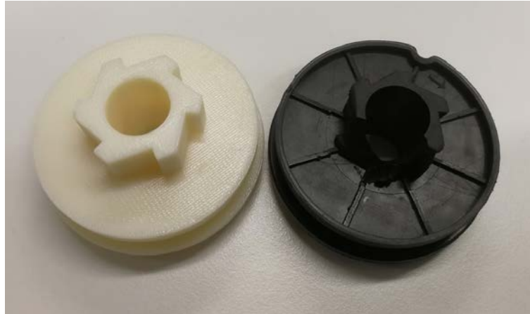
Kuva 20. Alkuperäinen ratas oikealla ja 3D-tulostettu ratas vasemmalla.
