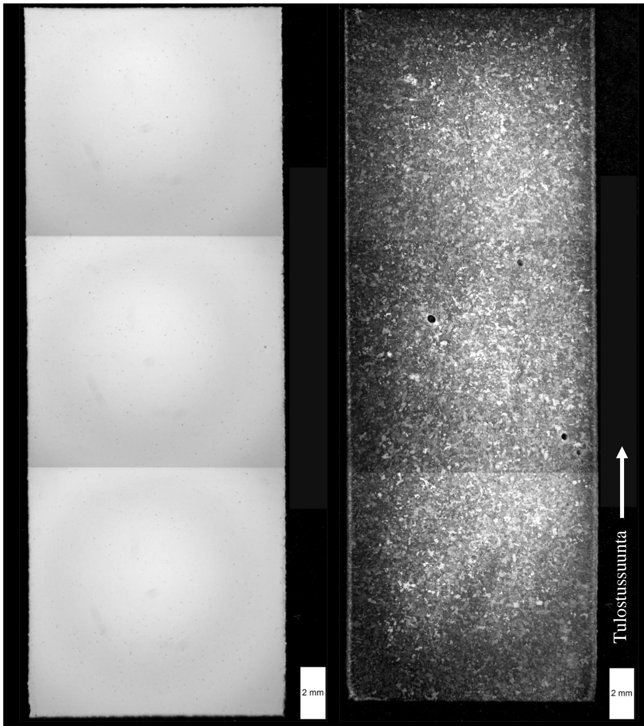
Kuva 2.2. 3D-tulostettu ja lämpökäsitelty (Jännitystenpoisto + HIP) Inconel 718 näyte a) ennen syövytystä, b) syövytyksen jälkeen.
