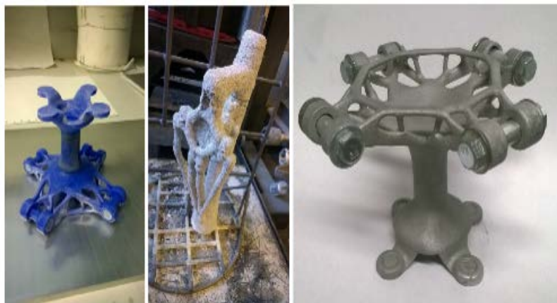
Kuva 17. Lapakeskiön tarkkuusvaluprosessi.
