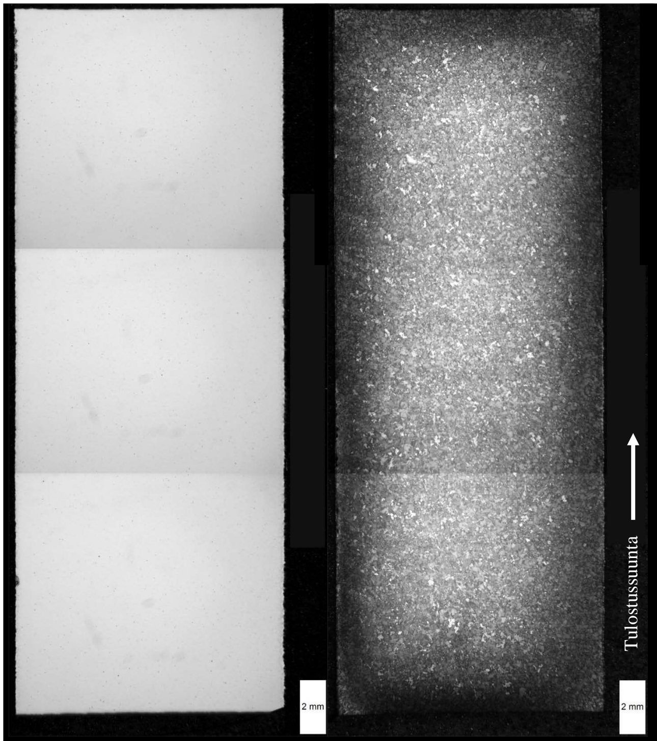
Kuva 2.3. 3D-tulostettu ja lämpökäsitelty (Jännitystenpoisto + HIP + Liuotushehkus + Erkautuskarkaisu) Inconel 718 näyte a) ennen syövytystä, b) syövytyksen jälkeen.
