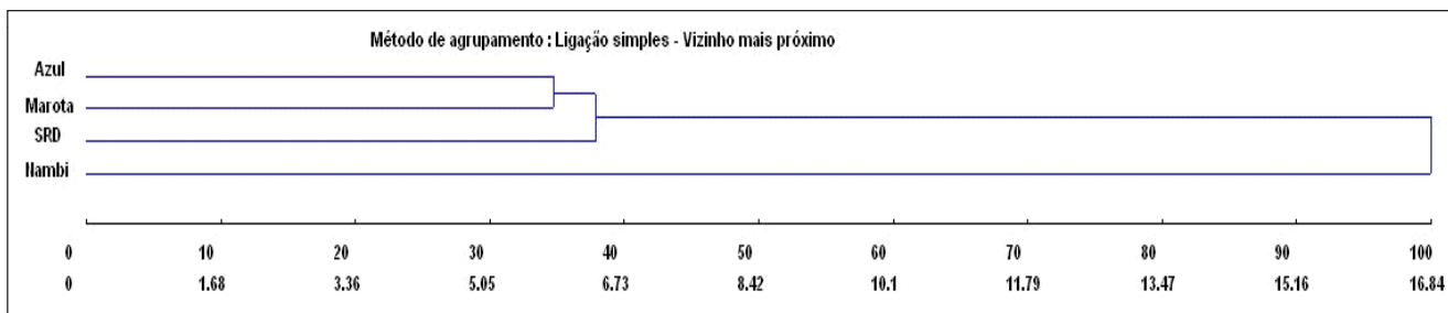
Fig. 1. Dendrograma pelo método do vizinho mais próximo utilizando as distâncias de Mahalanobis.
