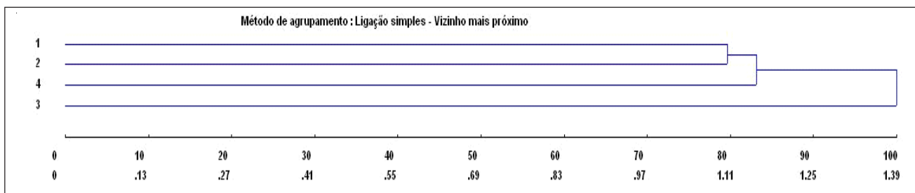
Fig. 2. Dendrograma pelo método do vizinho mais próximo utilizando as distâncias euclidianas médias. (1 = SRD, 2 = nambi, 3 = Azul, 4 = Marota).
