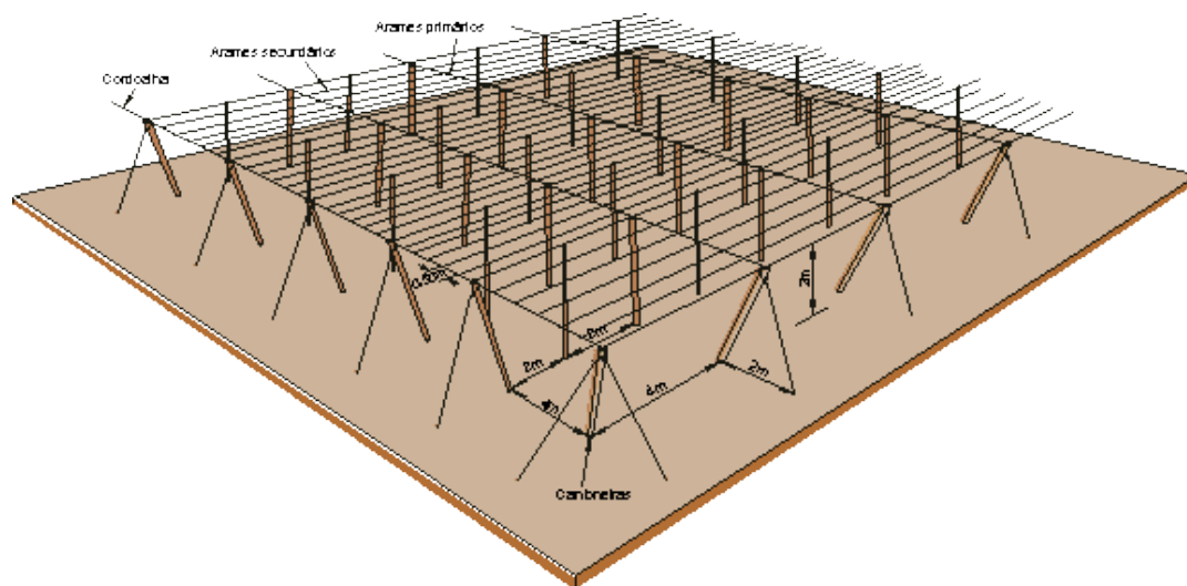
Fig. 1 - Vista geral de uma latada, com aramado, postes internos e externos
