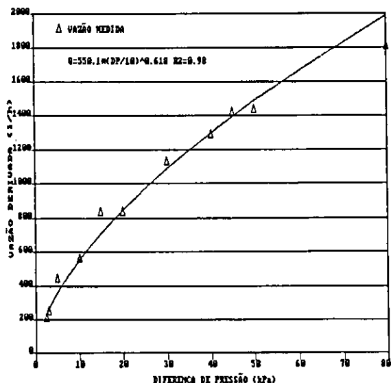
Figura 6 - Vazão derivada para o tanque de fertirrigação do CNPIL/EMBRAPA em função da diferença de pressão entre a entrada e a saída, gerada por registro, empregando-se conexões e mangueiras de 3/4".
