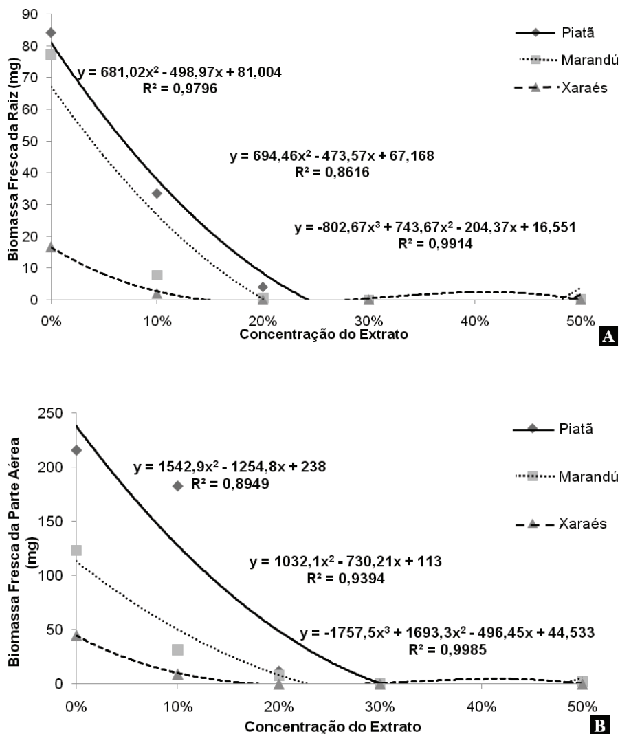
Figura 5. Biomassa fresca da raiz (A) e da parte aérea (B) de plântulas das braquiárias BRS Piatã, Marandú e Xaraés submetidas a diferentes concentrações de extrato de Brachiaria decumbens BRA001996. Regressão polinomial ( P < 0,05 ).
