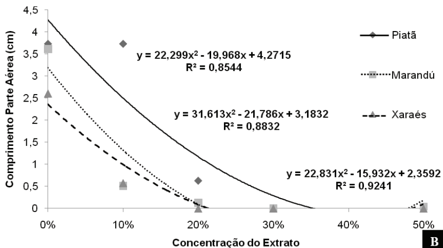
Figura 4. Comprimento da raiz (A) e comprimento da parte aérea (B) de plântulas das braquiárias BRS Piatã, Marandú e Xaraés submetidas a diferentes concentrações de extrato de Brachiaria decumbens BRAO01996. Regressão polinomial ( P < 0,05 ).
