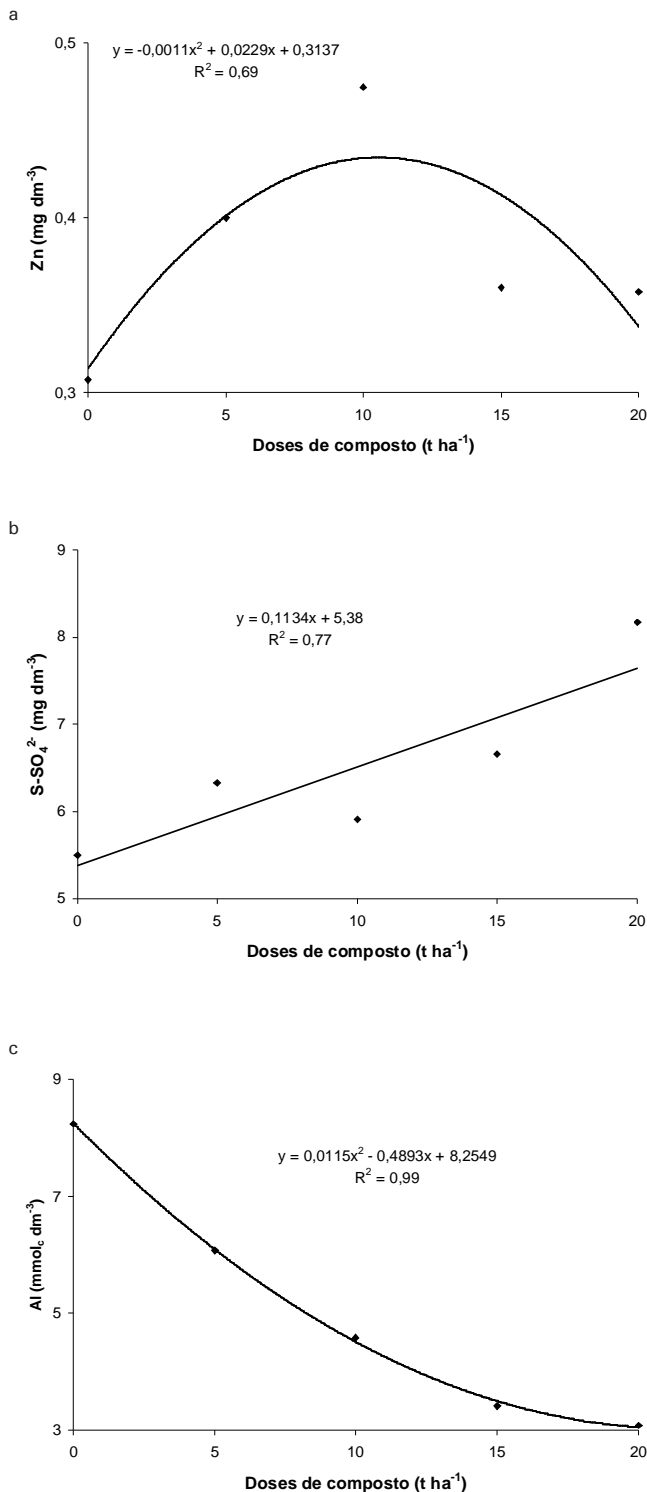
Figura 5. Efeito da aplicação composto orgânico de carcaça e despojo de abate de caprinos e ovinos nos valores Zn (a); S-SO 4 2- (b) e Al (c) no Latossolo.
