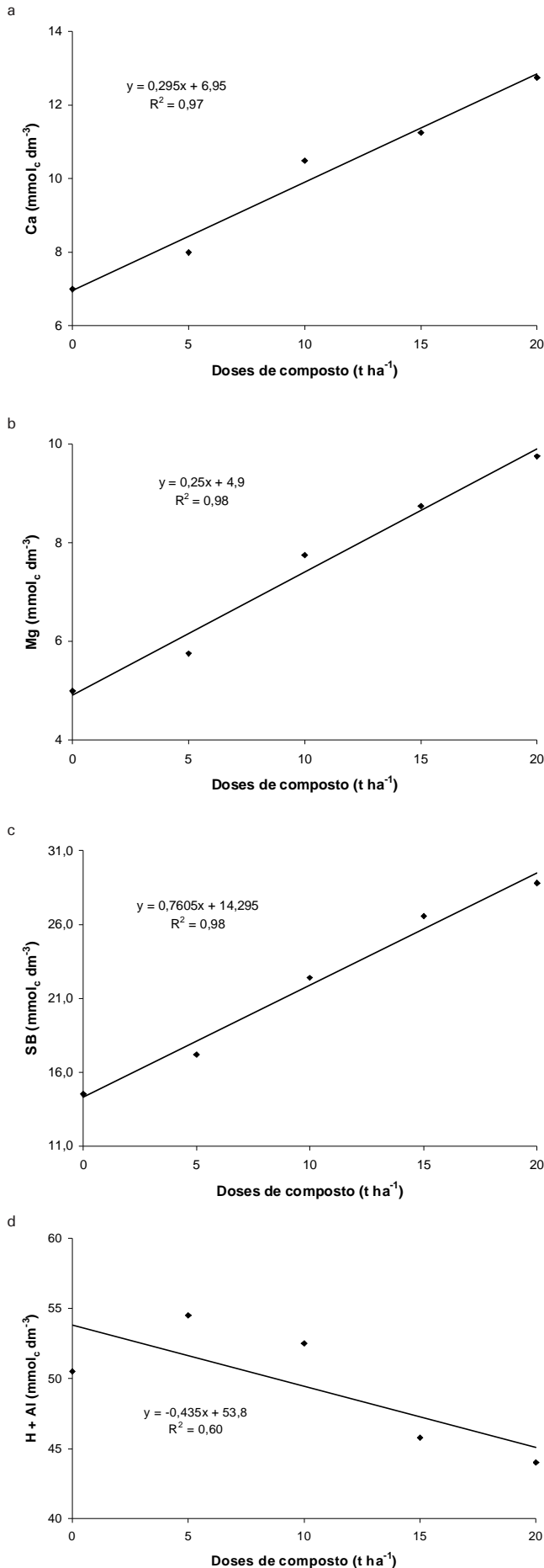
Figura 2. Efeito da aplicação do composto orgânico de carcaça e despojo de abate de caprinos e ovinos nos valores Ca (a); Mg (b); SB (c) e H + Al (d) do Latossolo.
