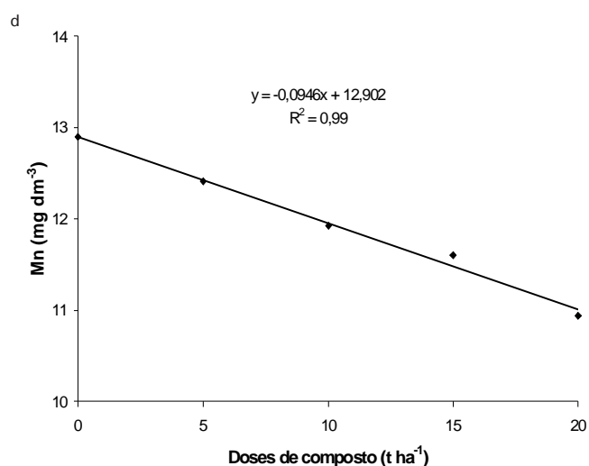
Figura 4. Efeito da aplicação do composto orgânico de carcaça e despojo de abate de caprinos e ovinos nos valores B (a); Cu (b); Fe (c) e Mn (d) no Latossolo.
