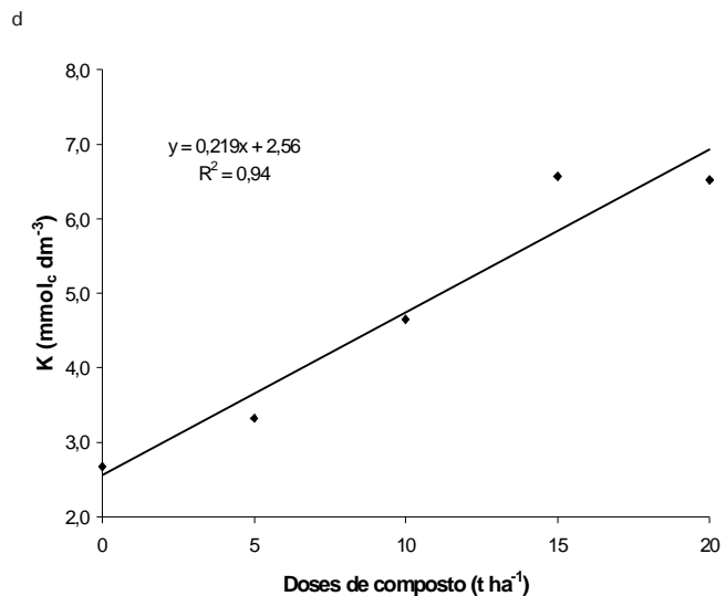
Figura 1abcd. Efeito da aplicação do composto orgânico de carcaça e despojo de abate de caprinos e ovinos nos valores pH (a); M.O. (b); P (c) e K (d) do Latossolo.
