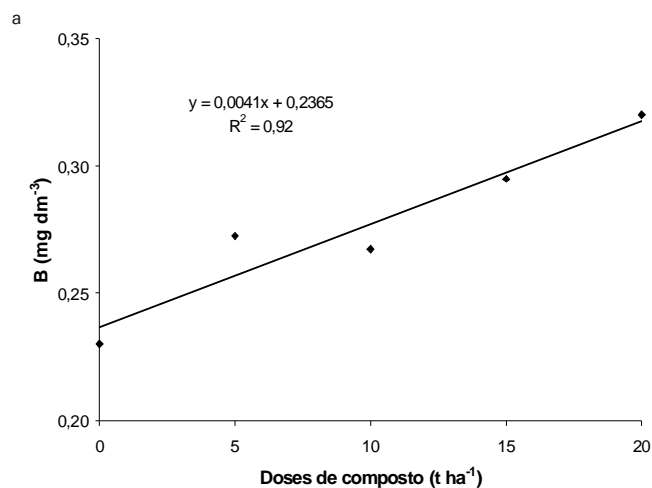
Figura 4. Efeito da aplicação do composto orgânico de carcaça e despojo de abate de caprinos e ovinos nos valores B (a); Cu (b); Fe (c) e Mn (d) no Latossolo.
