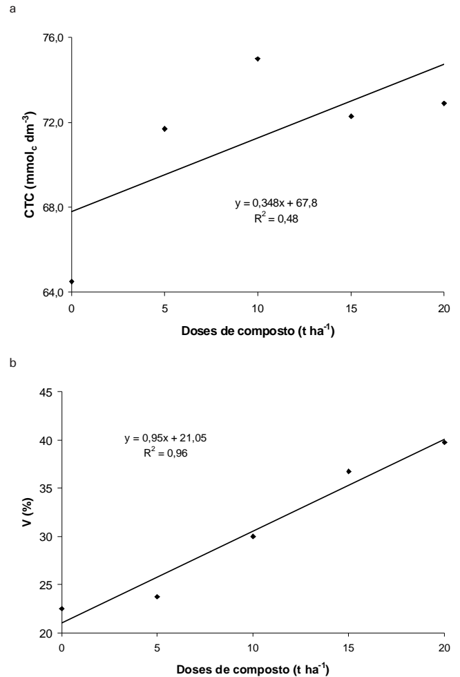
Figura 3. Efeito da aplicação de composto orgânico de carcaça e despojo de abate de caprinos e ovinos nos valores da CTC (a) e V (b) do Latossolo.
