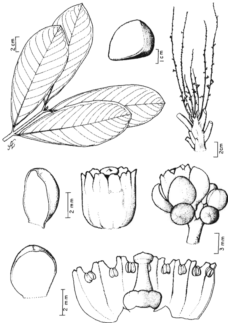
FIG. 5. Órgãos vegetativos e reprodutivos de Carapa guianensis Aubl. (Andiroba).
