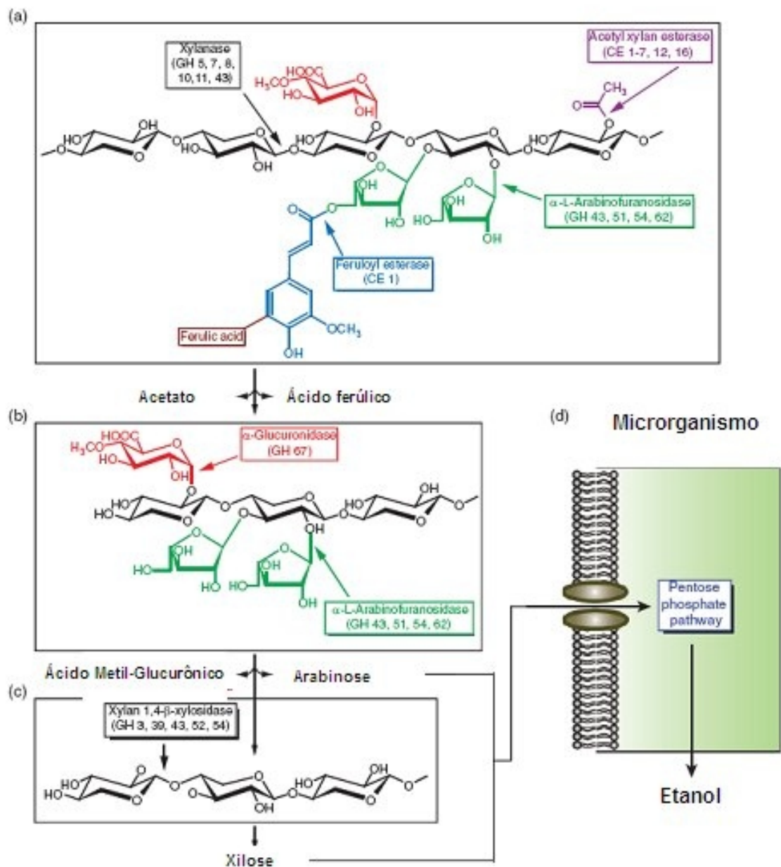
Fig. 6. Fluxograma esquemático representando a coordenação das enzimas xilanólíticas na desconstrução da hemicelulose visando à produção de biocombustíveis. (a) Xilanases, acetil-xilana-esterases e feruloil-esterases atuam em conjunto para produzir xilo-oligossacarídeos substituídos com a concomitante liberação de ácido ferúlico e ácido acético. (b) Arabinofuranosidas e glucuronidas, em seguida, liberam arabinose e ácido glucurônico destes xilo-oligossacarídeos. (c) As xilosidas convertem o xilo-oligossacarídeos em seus açúcares constituintes, xilose. (d) Microrganismos fermentativos selecionados podem finalmente utilizar os açúcares xilose e arabinose para produção de etanol (Adaptado de DODD; CANN, 2009).
