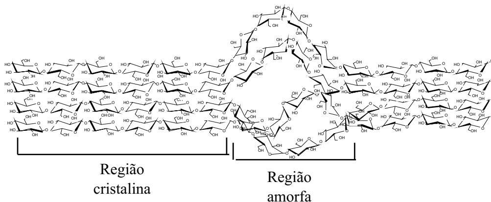
Fig. 2. Estrutura da celulose destacando as regiões cristalinas e amorfas.
