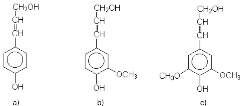
Fig. 4. Monômeros precursores da lignina (a) álcool trans-para-cumárico, (b) álcool trans-coneiférico e (c) álcool trans-sinapílico.
