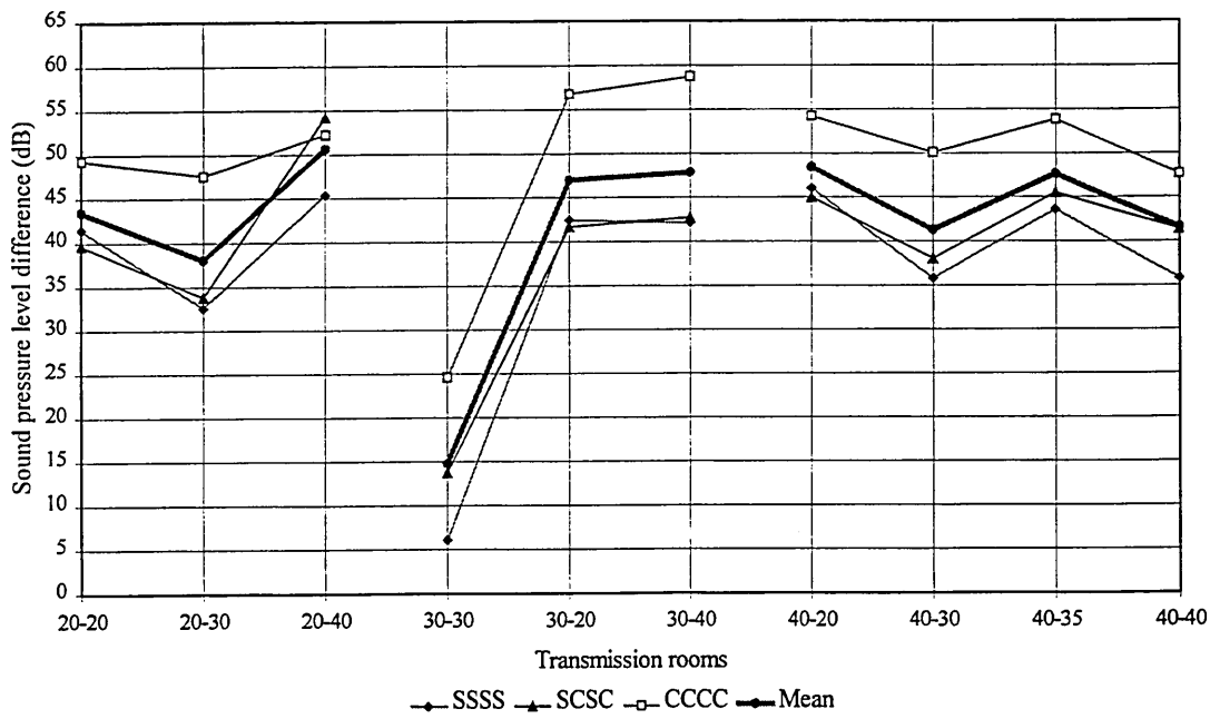
Figure10.11. 63Hz
