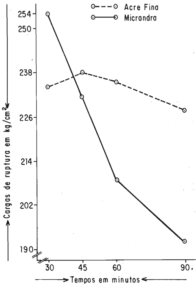
FIG. 1. Curvas de vulcanização.
