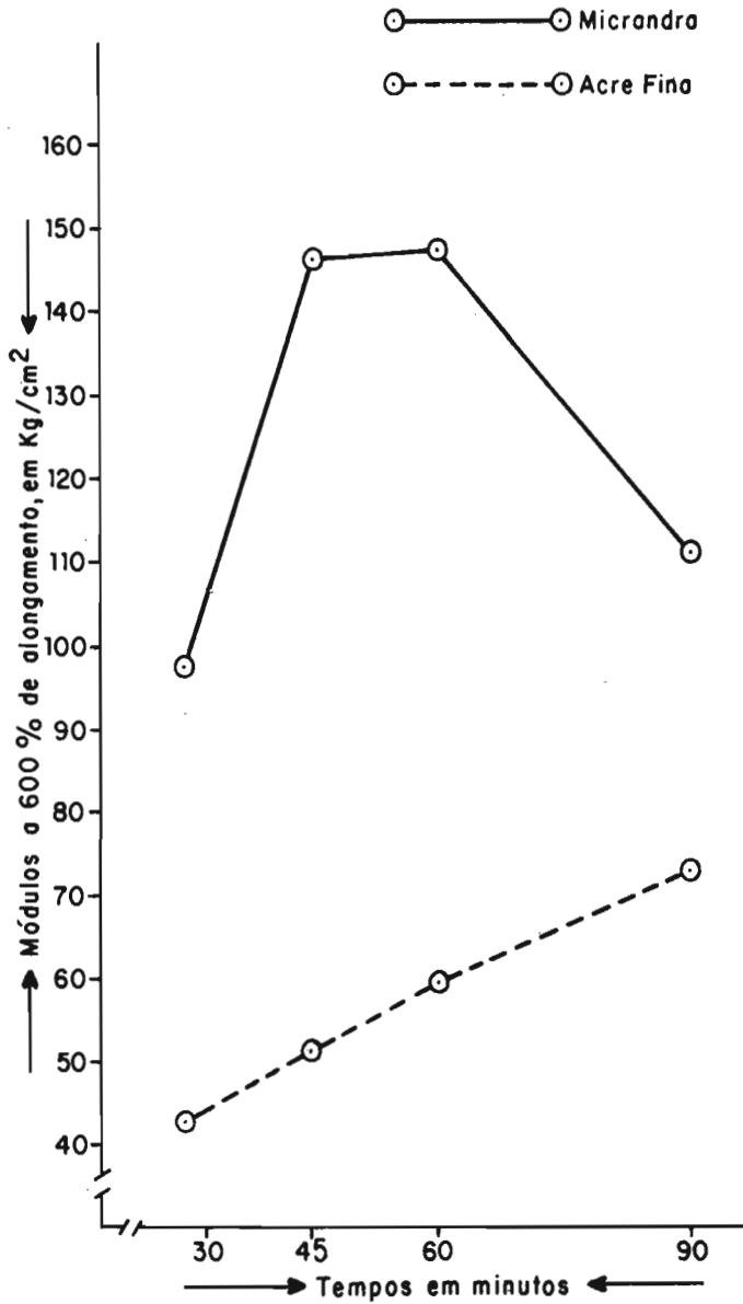
FIG. 2. Curvas de vulcanização.
