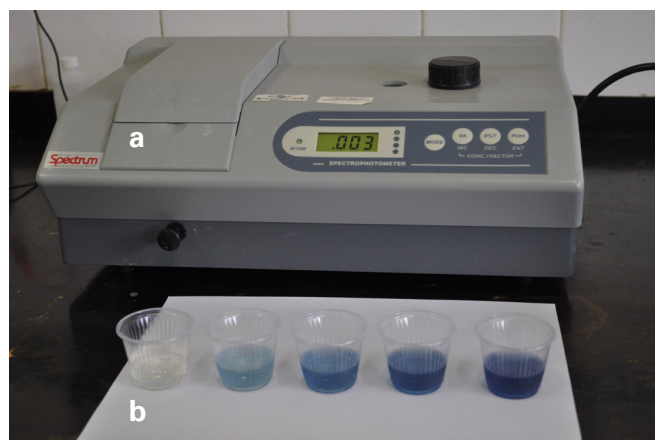
Figura 3. Espectrofotômetro UV/Visível utilizado para leitura colorimétrica do P na solução (a) e extratos de amostras de solos com variados teores de P na solução (b).
