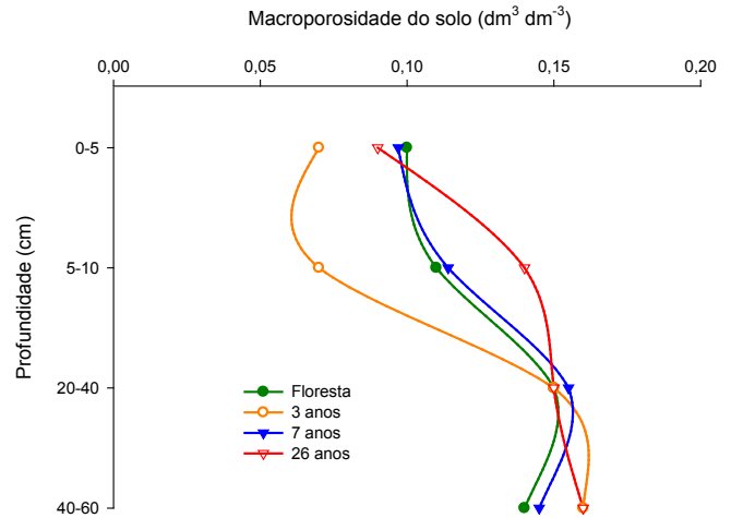
Figura 5. Macroporosidade do solo em floresta e em sistema de produção de café com diferentes tempos de aplicação de dejetos líquidos de suínos
