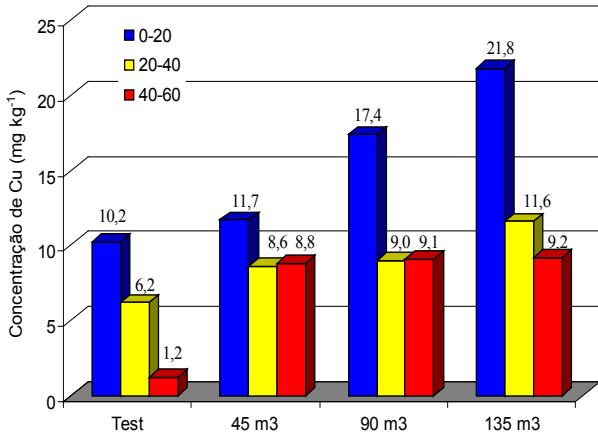
Figura 9. Concentração de Cu e Zn em Latosolo Vermelho após três anos sucessivos de aplicação de dejetos suínos
