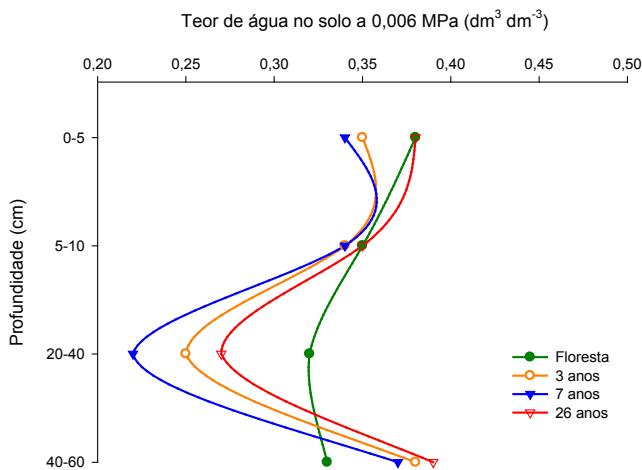
Figura 4. Teor de água retida no solo na tensão 0,006 MPa em floresta e em sistema de produção de café com diferentes tempos de aplicação de dejetos líquidos de suínos
