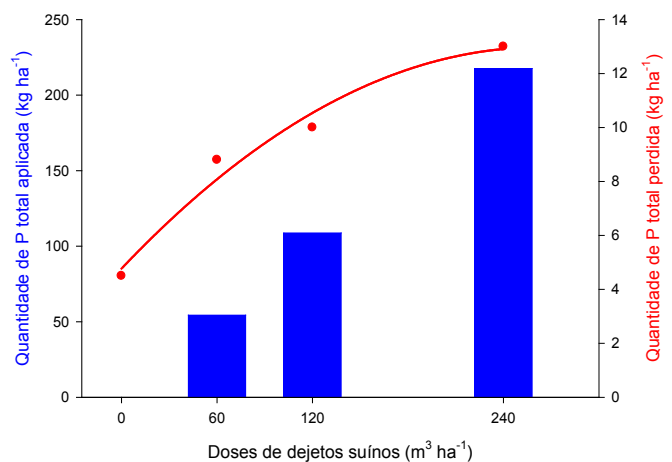
Figura 18. Quantidade de P aplicada e perdida por escoamento superficial em um ano agrícola em função da aplicação de DLS em Argissolo com 4% de declividade média, sob sistema plantio direto
