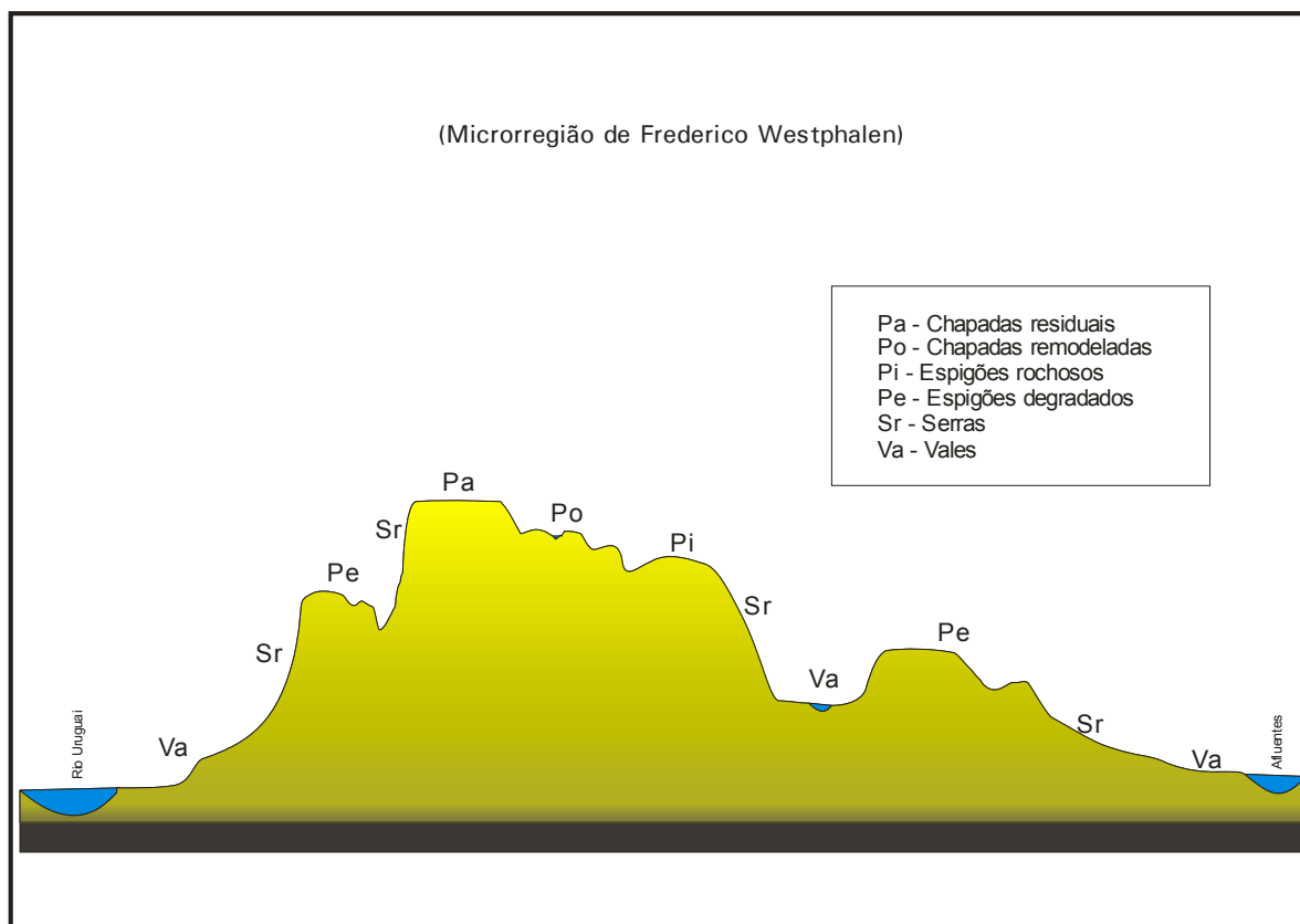
Fig 15: Secção transversal do relevo de municípios do Alto Uruguai, RS
