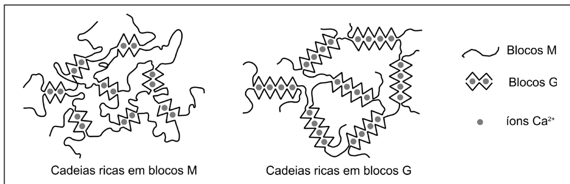
Figura 2. Redes de alginatos com blocos M e G, apresentando estruturas tipo "caixa de ovo" entre blocos G de cadeias adjacentes. (Fonte: BRODKORB, 2011).
