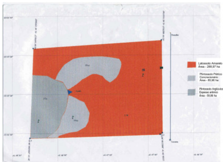
Mapa de Solos da Área da UEP/Parnaíba
