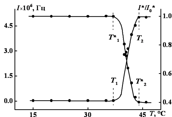
Р и с . 1. Зависимости I и I^*/I_0^* от T для раствора ПИ- g -ПДМАЭМА рН = 11.9 ( I_0^* - величина оптического пропускания при комнатной температуре)
