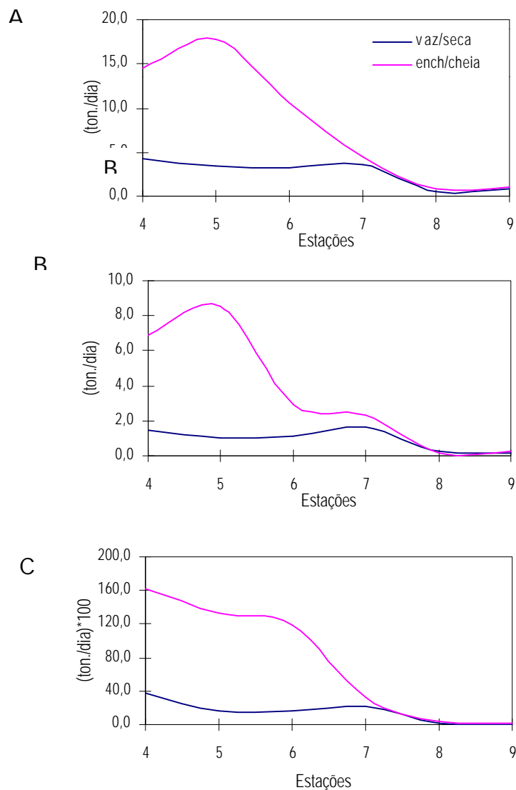
Fig. 3. Cargas médios de NT(A), PT(B) e SST(C) (ton./dia) nos trechos médio e inferior do rio Taquari, no período de dezembro/95 a maio/97.
