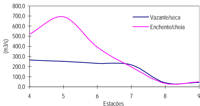
Fig. 2. Vazão ( \text{m}^3/\text{s} ) média do rio Taquari nas estações 4 a 9, nas fases de vazante/seca e enchente/cheia dos anos de 1995 a 1997.
