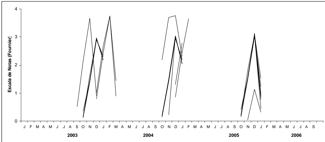
Figura 5. Períodos de ocorrência e percentagem de árvores de Ocotea porosa , em estágio de frutos novos, em quatro anos consecutivos. Segundo escala de notas (FOURNIER, 1974). Colombo, PR. 2003-2006.
