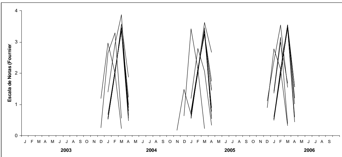
Figura 7. Períodos de ocorrência e percentagem de árvores de Ocotea porosa , em estágio de frutos maduros, em quatro anos consecutivos. Segundo escala de notas (FOURNIER, 1974). Colombo, PR. 2003-2006.
