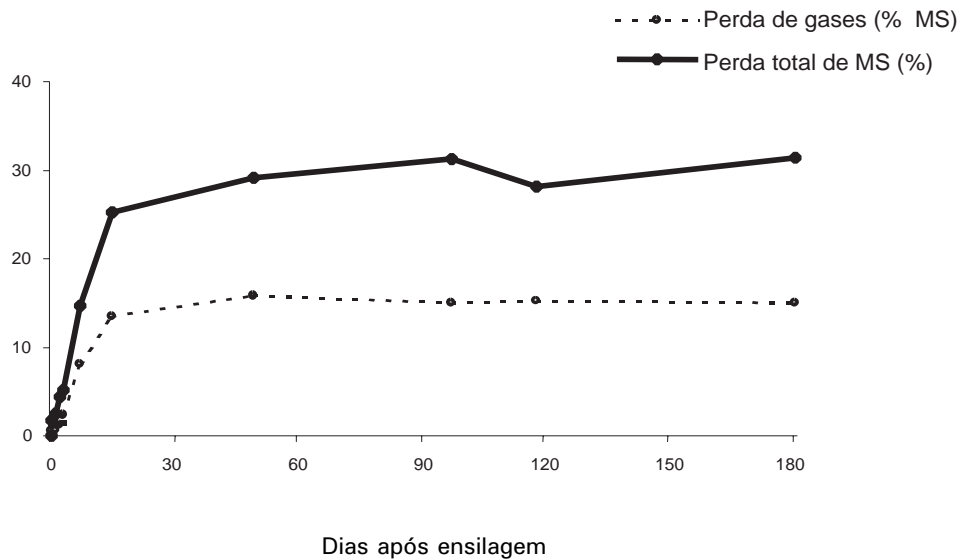
Figura 2 - Evolução temporal da perda de gases e da perda total de matéria seca (MS) em silagem de cana-de-açúcar.
