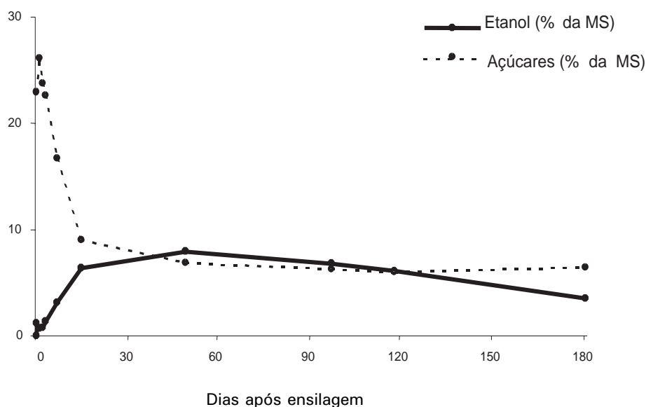
Figura 1. Evolução temporal da concentração de etanol e de açúcares na matéria seca (MS) de silagem de cana-de-açúcar.
