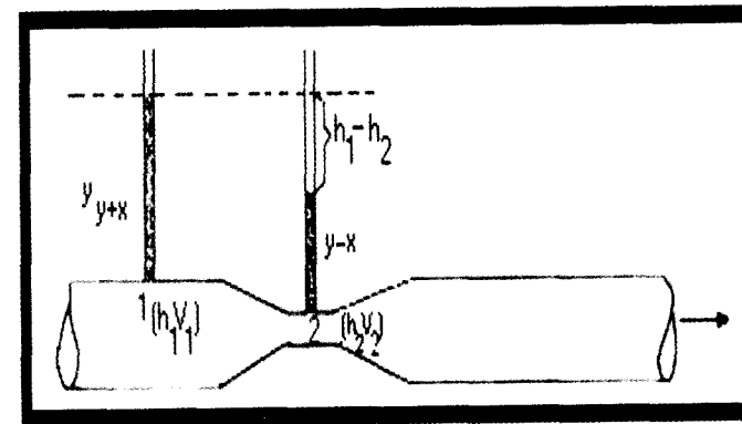
Fig. 6. Detalhe do sistema hidráulico de um venturi Fonte: Costa & Brito, 1994.
