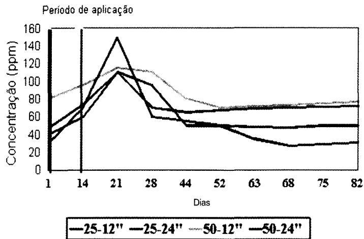
Fig. 18. Evolução da concentração de potássio na solução do solo. Fonte: PAR/CSIC (1999).
