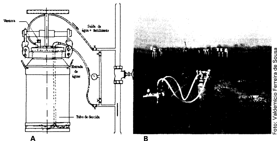
Fig. 9. Esquema do tanque de derivação de fluxo (A) e detalhe de instalação no campo (B)
