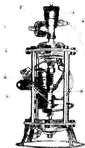
Fig. 11. Bomba injetora de fertilizantes de ação hidráulica por diafragma (TMB).
