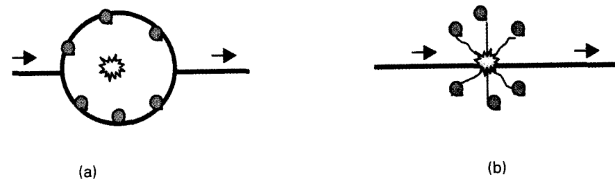
Fig. 2. Disposição mais recomendada dos gotejadores em culturas de médio e grande porte.
