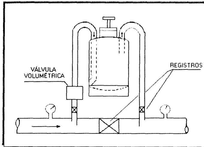
Fig. 8. Esquema de um tanque de derivação de fluxo.
