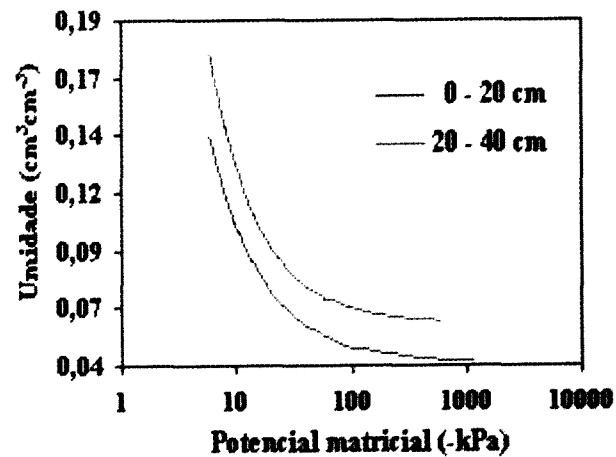
Fig. 5. Curva de retenção de água no solo.
