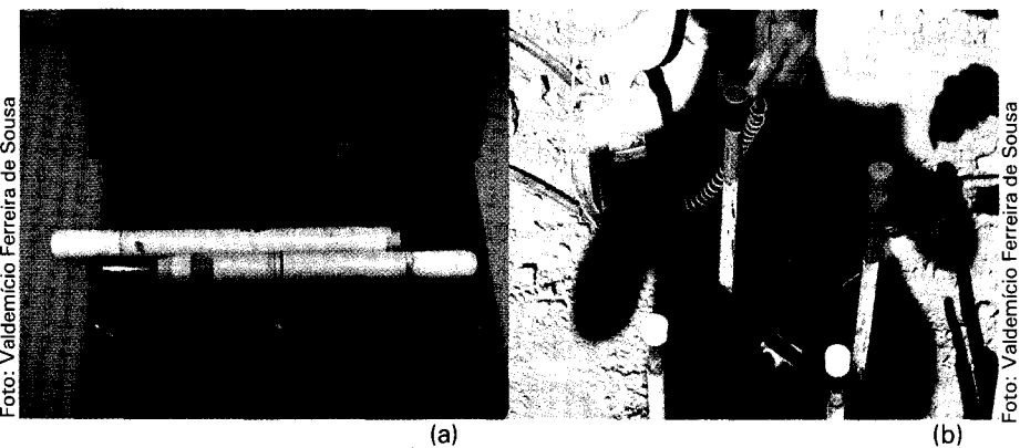
Fig. 4. Detalhes do tensiômetro confeccionado para utilização de leitura digital (a) e do leitor digital do potencial (tensímetro) no momento da leitura (b).
