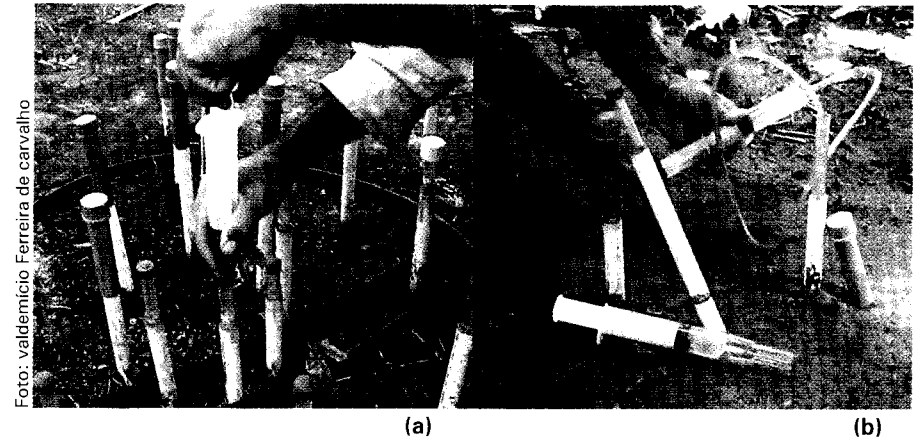
Fig. 21. Procedimento da extração de solução do solo, utilizando-se extratores de cápsula porosa e seringa descartável.
