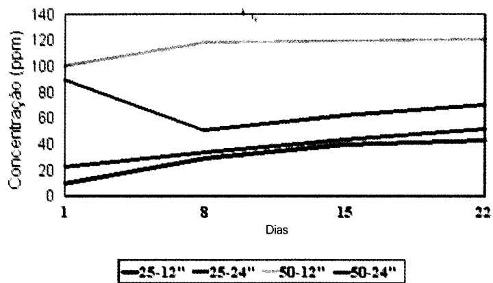
Fig. 17. Evolução da concentração de N(NO 3 ) na solução do solo Fonte: PAR/CSIC (1999).
