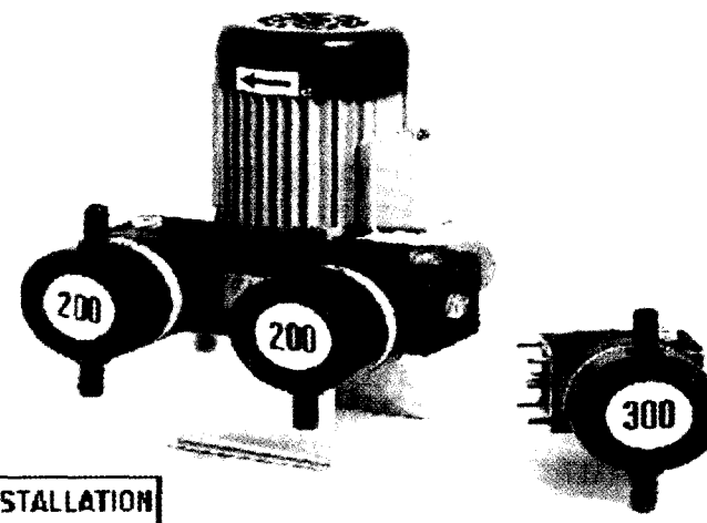
Fig. 13. Bomba injetora de fertilizantes de acionamento elétrico com diferentes módulos de injeção. "Fonte: ITC (2000?)."
