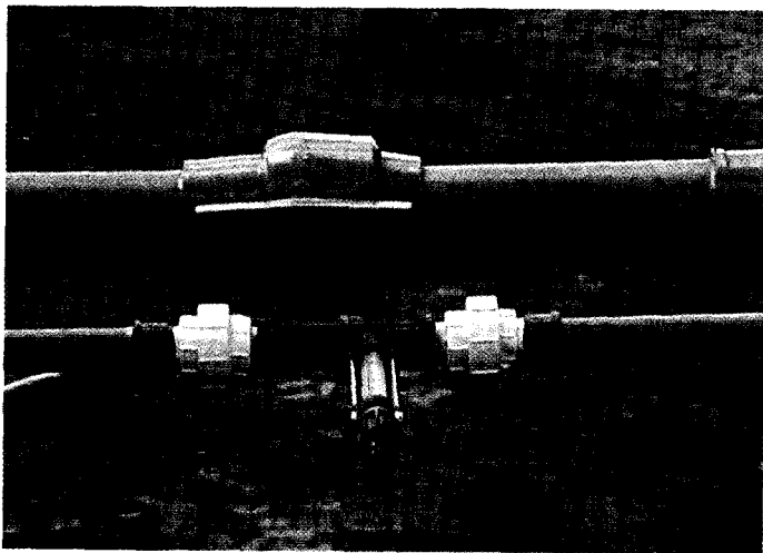
Fig. 7. Injetor venturi instalado em esquema "by pass".
