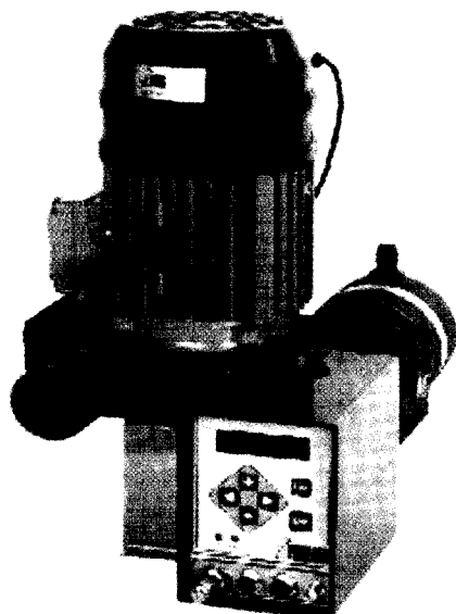
Fig. 23. Leitor de condutividade elétrica, pH e vazão, acoplado a uma bomba elétrica para injeção de fertilizantes Fonte: ITC (2000?).
