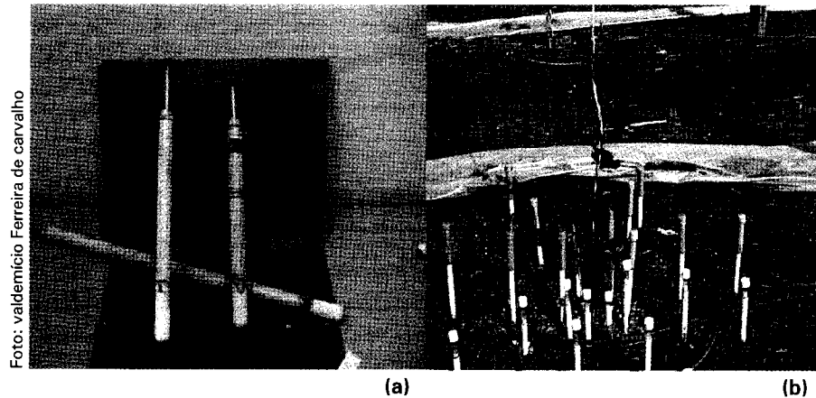
Fig. 20. Extratores de solução. Detalhe de confecção (a) e instalado no solo (b). Fonte: Sousa & Andrade Júnior (1999).
