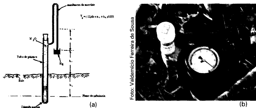
Fig. 3. Tensiômetros com manômetro de mercúrio (a) e com vacuômetro de bourdon (b).
