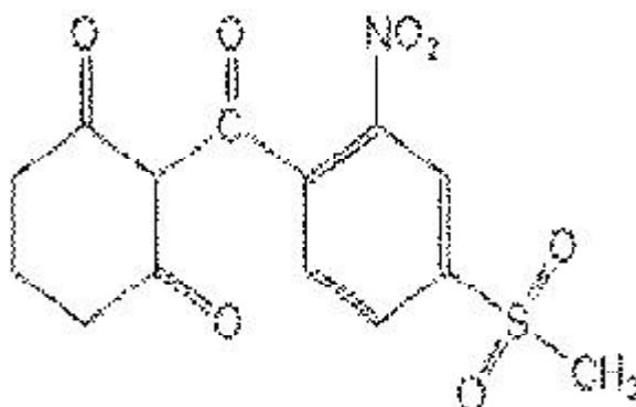
Figura 1. Fórmula química de mesotrione.
