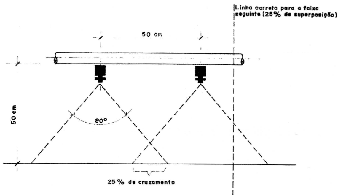
FIGURA 5 - Posição correta dos BICOS e cruzamento adequado dos jatos
