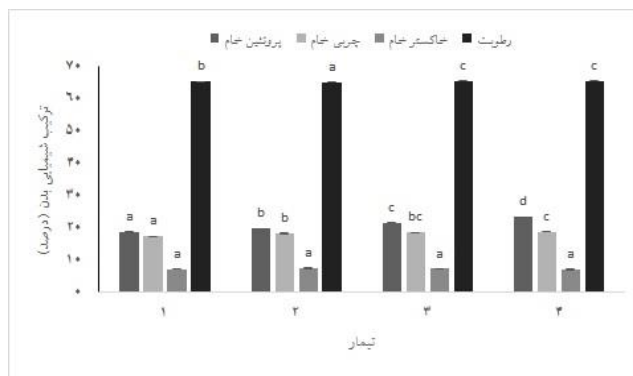
نمودار ۱. ترکیب شیمیایی لاشه کفال ماهی در تیمارهای مختلف در پایان دوره آزمایش (روز ۶۲) (میانگین \pm خطای معیار) ( n=9 ) وجود حروف غیر همسان در هر ردیف نشانه اختلاف معنی دار است ( P<0/05 ).
