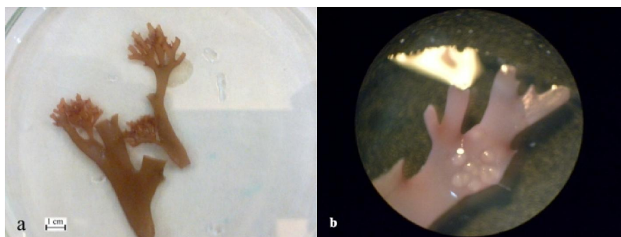
شکل ۴: شکل ظاهری گامتوفیت ماده (a) و نمایش سطحی از زوائد سیستوکارب نیمه کروی بالغ با استفاده از استریو میکروسکوپ (b)
