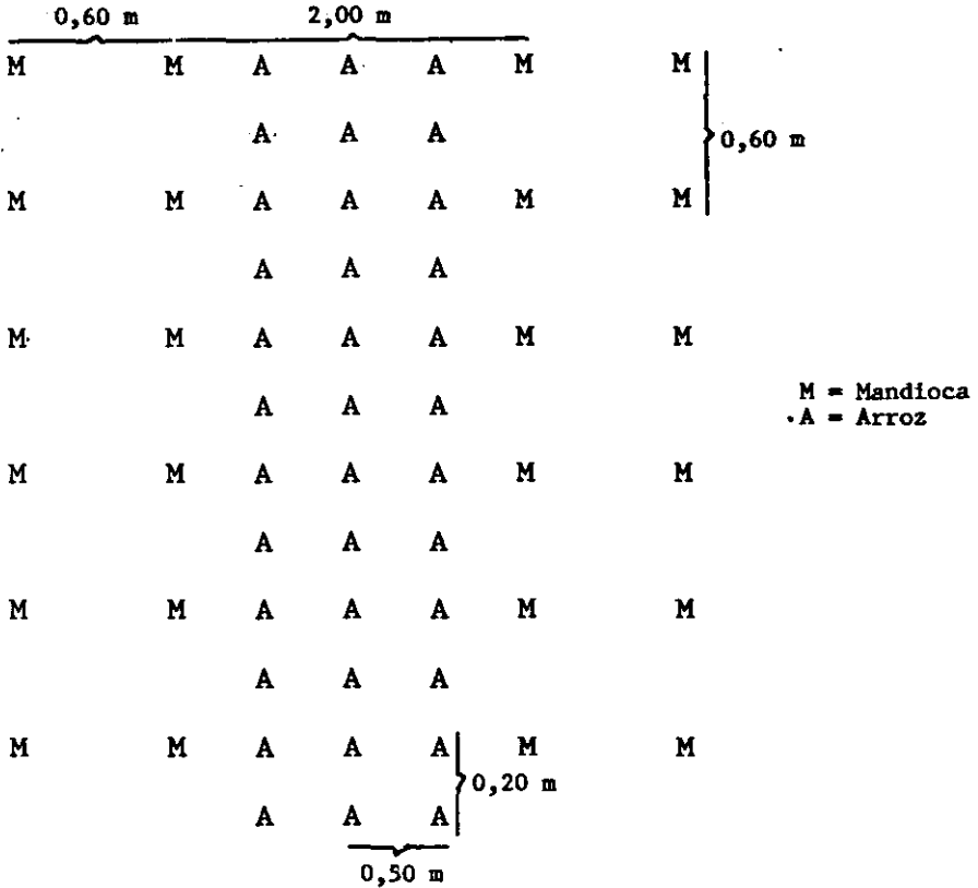
FIG. 2. Arranjo espacial do consórcio mandioca em fileiras duplas com três fileiras de arroz.
