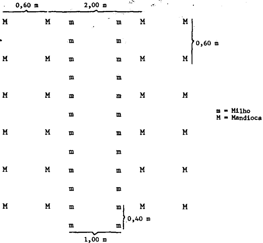
FIG. 3. Arranjo espacial do consórcio mandioca em fileiras duplas com duas fileiras de milho
