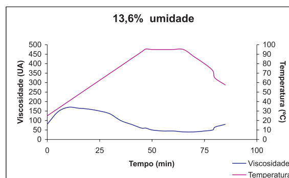
Fig. 1. Viscosidade de pasta de extrusado de fubá com 13,6 % de umidade.
