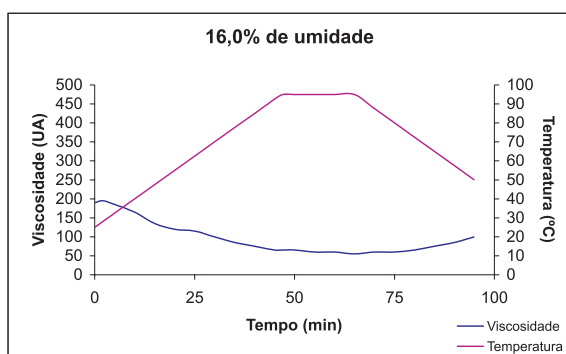
Fig. 2. Viscosidade de pasta de extrusado de fubá com 16,0 % de umidade.
