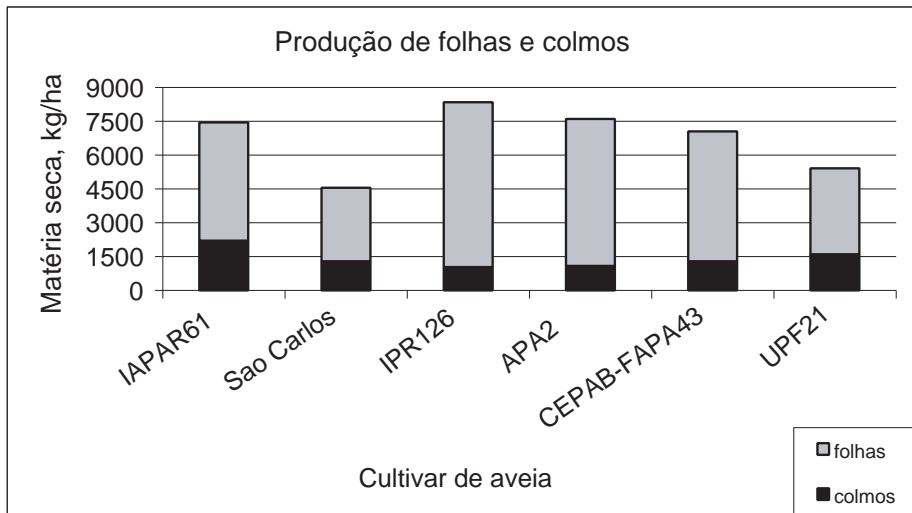
Figura 1. Proporção de folhas e de colmos acumulados na estação de crescimento, para cada cultivar de aveia forrageira.
