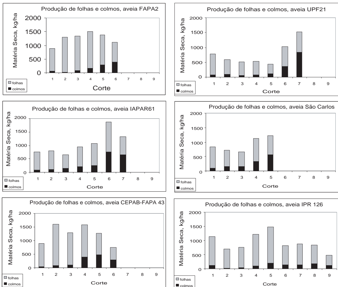
Figura 2. Proporção na matéria seca de folhas e de colmos ao longo dos cortes em seis cultivares de aveia forrageira.
