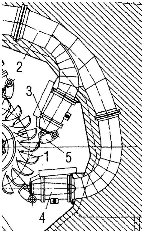
Abbildung 2 Schnitt einer Pelton-turbine, 1 Laufrad, 2 Ringleitung, 3 Düse, 4 innenregulierte Düsennadel, 5 Strahlableiker, [4, p. 98]
