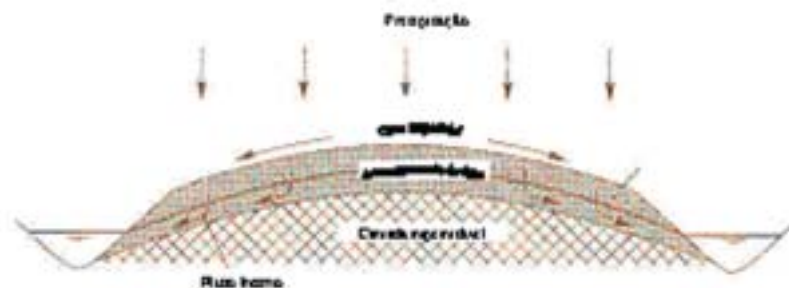
Figura 1a - Drenagem superficial de água no solo em áreas de cavilhão (adaptado de Smedema e Rycroft, 1983)
