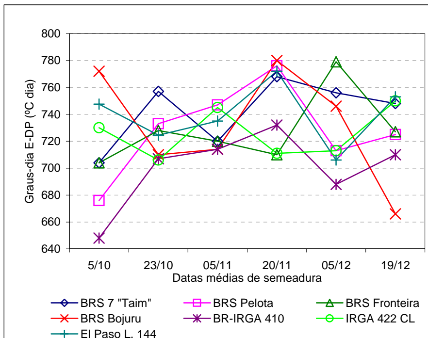
Figura 9. Graus-dia médios da emergência à diferenciação da panícula (°C dia), de sete cultivares de arroz irrigado, de ciclo Médio, em seis datas médias de semeadura, nas safras de 2004/05 a 2007/08, em Capão do Leão, RS.
