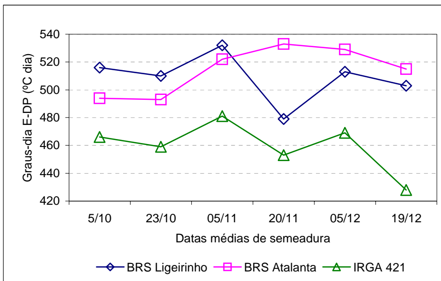
Figura 7. Graus-dia médios da emergência à diferenciação da panícula ( ^{\circ}\text{C dia} ), de três cultivares de arroz irrigado, de ciclo Muito Precoce, em seis datas médias de semeadura, nas safras de 2004/05 a 2007/08, em Capão do Leão, RS.
