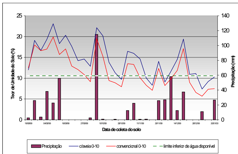
Figura 2. Umidade do solo na profundidade de 10 a 20 cm em pomar de pessegueiro cv. Cerrito, cultivado com aveia preta e no sistema convencional: limite inferior de água e precipitação pluviométrica. Embrapa Clima Temperado, Pelotas/RS, 2005.
