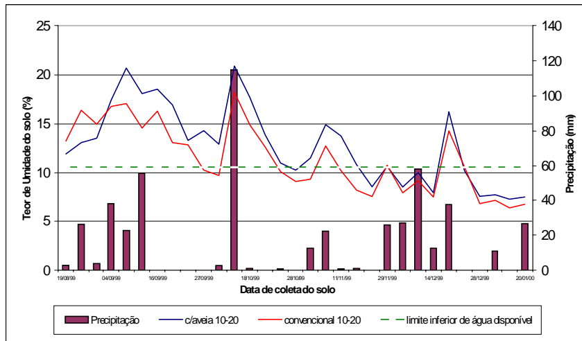
Figura 1. Umidade do solo na profundidade de 0 a 10 cm, em pomar de pessegueiro cv. Cerrito, cultivado com aveia preta e sistema convencional: limite inferior de água e precipitação pluviométrica. Embrapa Clima Temperado, Pelotas/RS, 2005.
