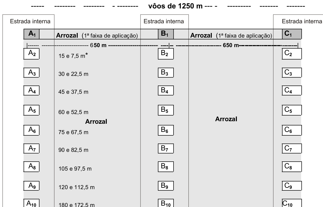
Figura 1. Disposição das fileiras de bandejas plásticas (A, B e C) em arrozal submetido à aplicação do inseticida carbofuran granulado por via aérea. A posição das bandejas A 1 , B 1 e C 1 corresponde ao centro da primeira faixa de aplicação. *Distância do centro e da borda da faixa de aplicação, respectivamente. Embrapa Clima Temperado, Pelotas - RS, 2002.
