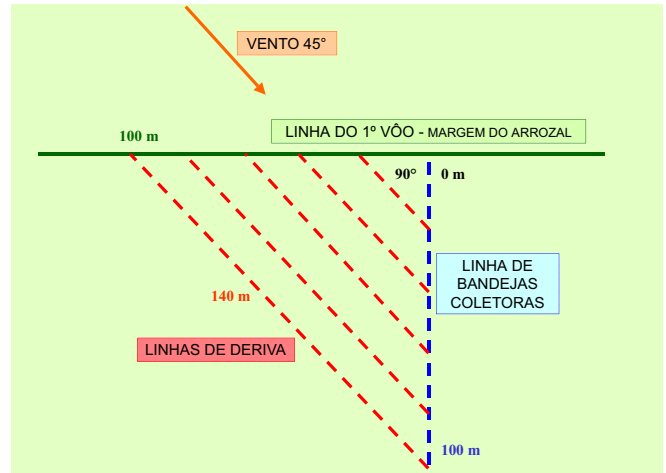
Figura 3. Diagrama das linhas, de vôo, das bandejas coletoras, da direção do vento e da deriva. Pelotas-RS, 2002.
