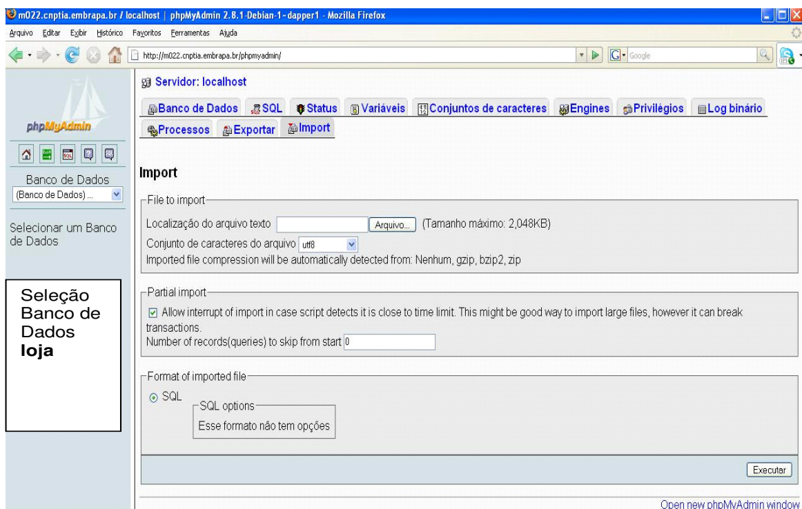
Fig. 2. Importação estrutura do banco de dados.
