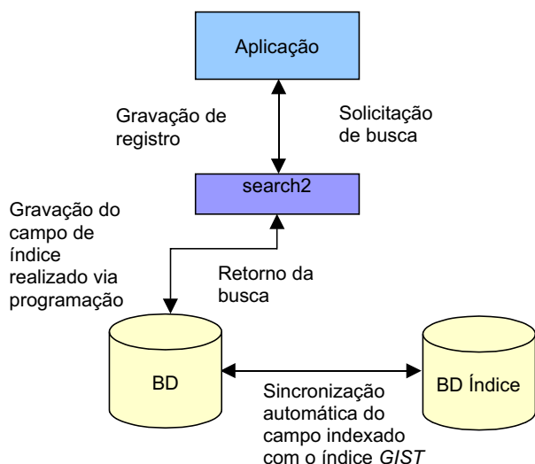
Fig. 1. Arquitetura Tsearch2 para PostgreSQL.
