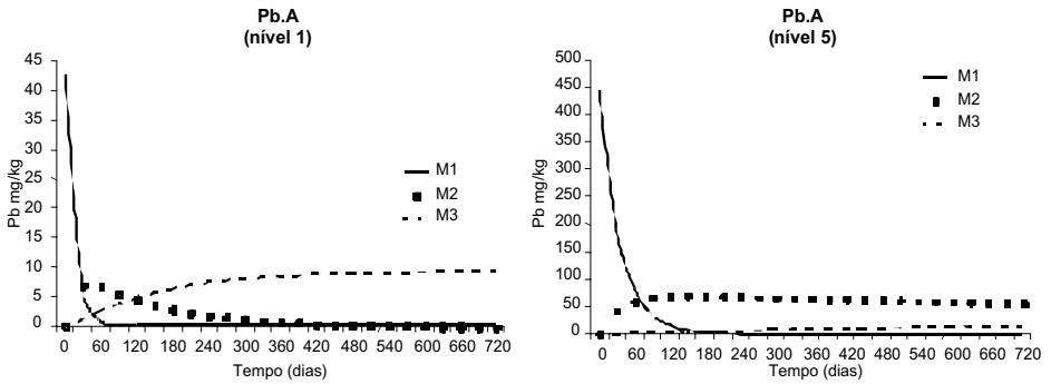
Fig. 6. Modelo de Transferência de Metal Pesado para o Pb em solos A, sob adubação de 0 t.ha -1 de CL (nível 1) e de 90 t.ha -1 de CL (nível 5).
