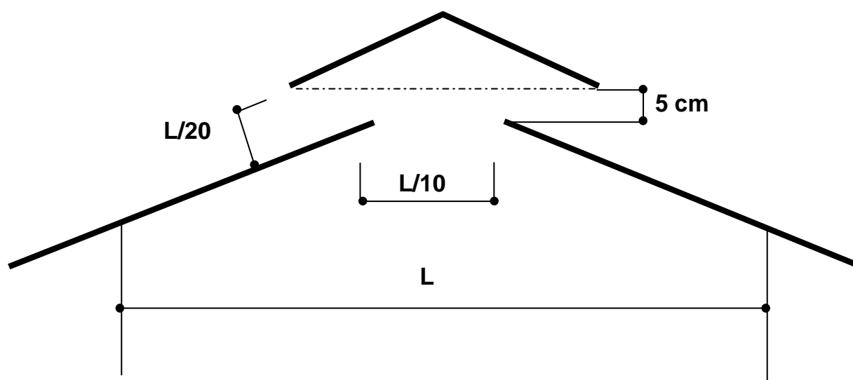
FIGURA 1 – Esquema para determinação das dimensões do lanternim.
