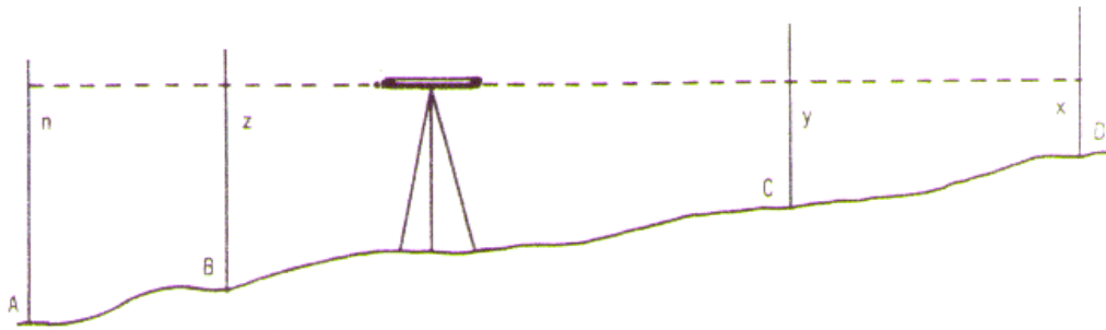
Fig. 6.11. Nivelamento simples com nível de luneta
