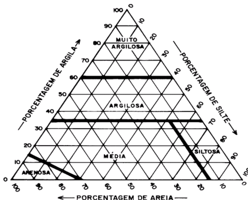
Fig. 2.3. Triângulo de agrupamento textural. Fonte: EMBRAPA, 2006.
