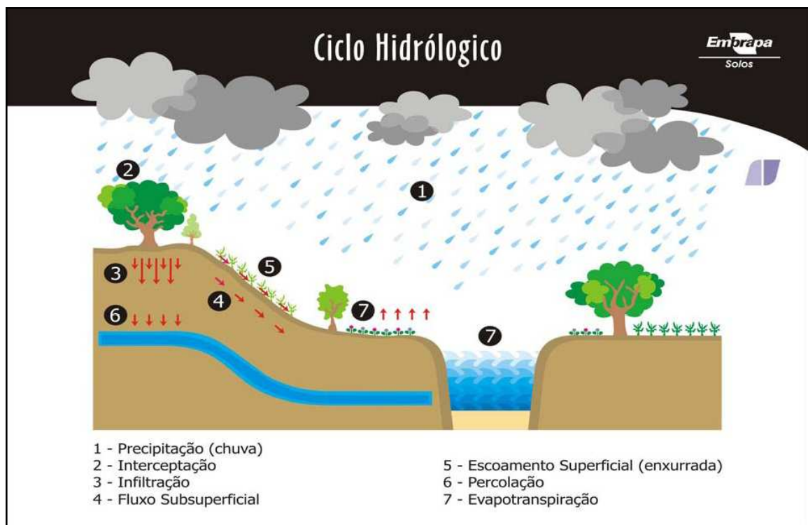
Fig. 5.17. Ciclo Hidrológico apresentando a água nas diversas fases e situações.
