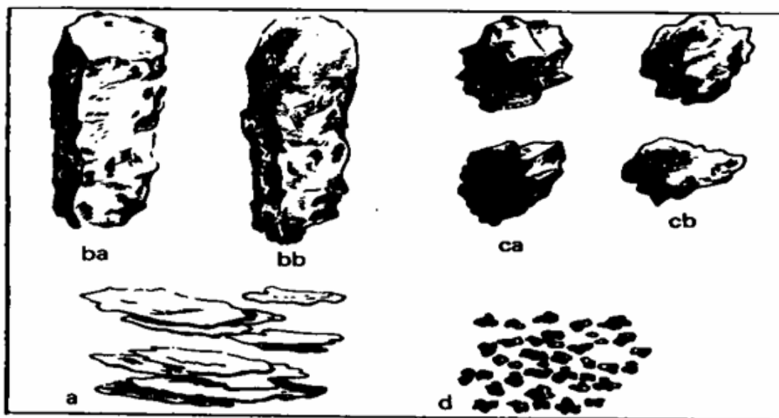
Fig. 2.4. Tipos de estrutura: (a) laminar; (bb) prismática; (ba) colunar; (ca) blocos angulares, (cb) blocos sub angulares; (d) granular.
