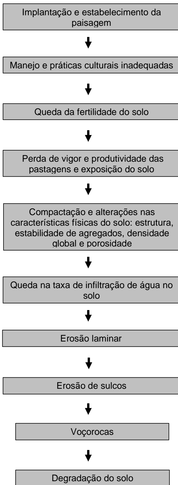
Fig.7.7. Seqüência típica de um processo de degradação da pastagem e conseqüentemente do solo:
