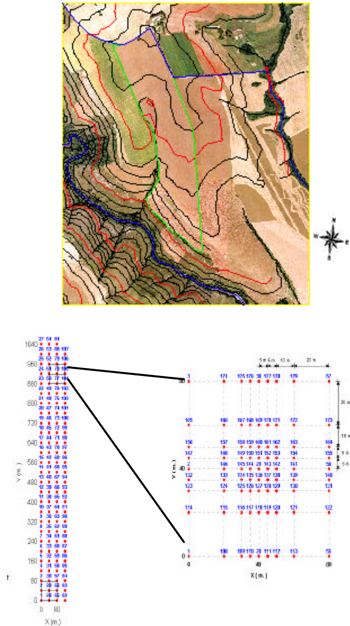
Fig. 1. Ortofoto da área de estudo (destacada em verde) e esquema das malhas de amostragens adotadas.
