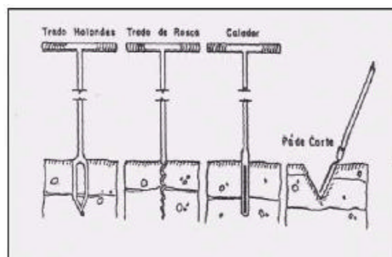
Figura 3. Equipamentos manuais utilizados para a amostragem de solos.
