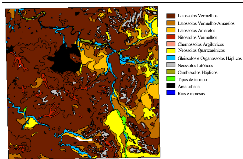
Fig. 3. Distribuição espacial das classes de solos, ao nível categórico de subordens, da quadrícula de Ribeirão Preto-SP (Oliveira & Prado, 1987; Embrapa-CNPS, 1999).
