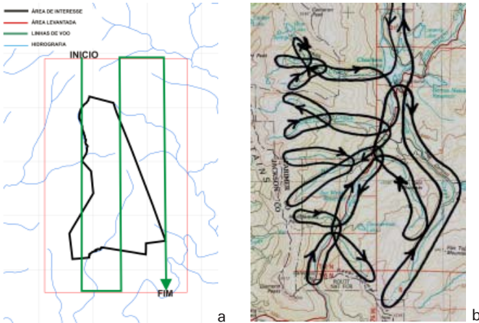
Fig. 9. Planejamento do vôo em (a) grid ou (b) do tipo "contour".
