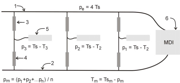
Fig. 3 - Esquema do sistema medial de leitura da tensão média ( T_m ) da água no solo com sensores Irrigas. 1- linha de entrada de ar na pressão p_e , 2- linha de leitura com a pressão de ar média ( p_m ) dos sensores, 3 - restrição ou capilar de entrada, 4 - restrição de saída, 5 - sensor Irrigas instalado no solo, 6- Instrumento com fonte de ar de pressão ajustada e leitor de pressão, T_s - tensão crítica de sorção, p_1, p_2 \dots p_n pressões de ar nos respectivos sensores Irrigas, T_1, T_2 \dots T_n as tensões de água do solo na vizinhança de cada sensor Irrigas.
