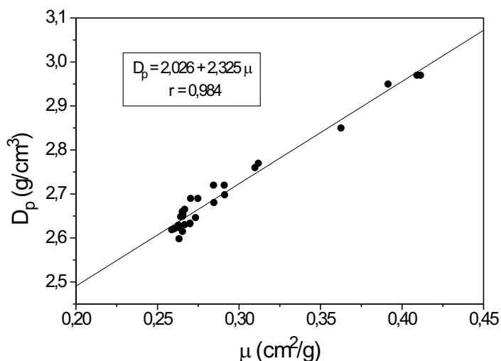
Figura 4. Correlação experimental entre o coeficiente de atenuação e a densidade das partículas de alguns solos.
