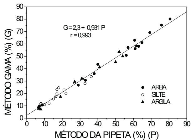
Figura 6. Comparação entre o método de atenuação da radiação gama e da Pipeta.
