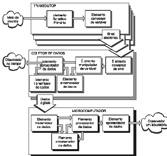
Figura 1 - Configuração de um Sistema de Aquisição de Dados normalmente encontrado em coletores de dados (topologia de transdutores em estrela).
